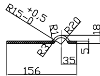
A-A (旋转)
