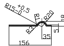
B-B (旋转)
