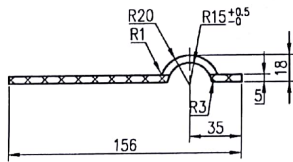
A-A (旋转) 1:2
