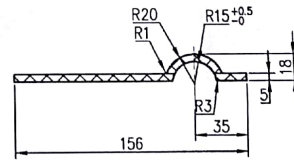
B-B (旋转) 1:2
